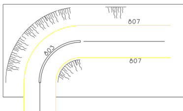
תרשים מס' 1 (809 - 801): סימון עקרוני של קו רצוף כפול 803 בעקומה אופקית.
