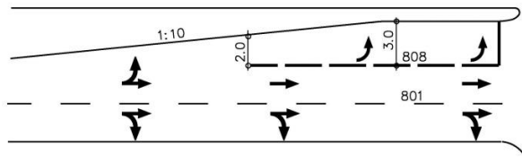
תרשים מס' 23 (801 - 809): סימון 808 "מלבנים קצרים" להפרדה בין נתיב המיועד לפניה שמאלה ובין הנתיבים לנסיעה ישר (מתוך מ.מ. 1)
