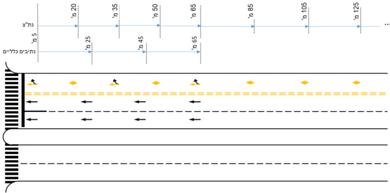
תרשים מס' 7 (501 - 504): מרווחים בין חיצים ומעויינים בדרך עירונית
