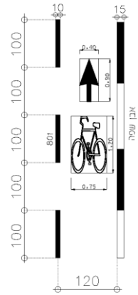
בתנועה חד סטרית בנתיב עם כוון התנועה
