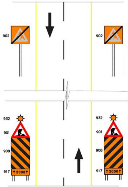
תרשים מס' 2 (901-902): התמרורים המוצבים בשער הכניסה וביציאה ממנו, ב"אתר עבודה" (מתוך מ.מ. 43).
