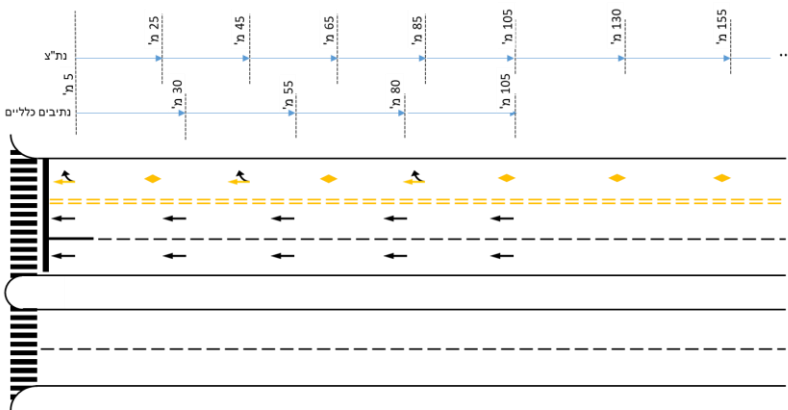
תרשים מס' 8 (501 - 504): מרווחים בין חיצים ומעויינים בדרך לא עירונית
