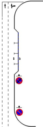
ביטול איסור העצירה עקב שינוי החתך (תוספת מפרץ חניה).
